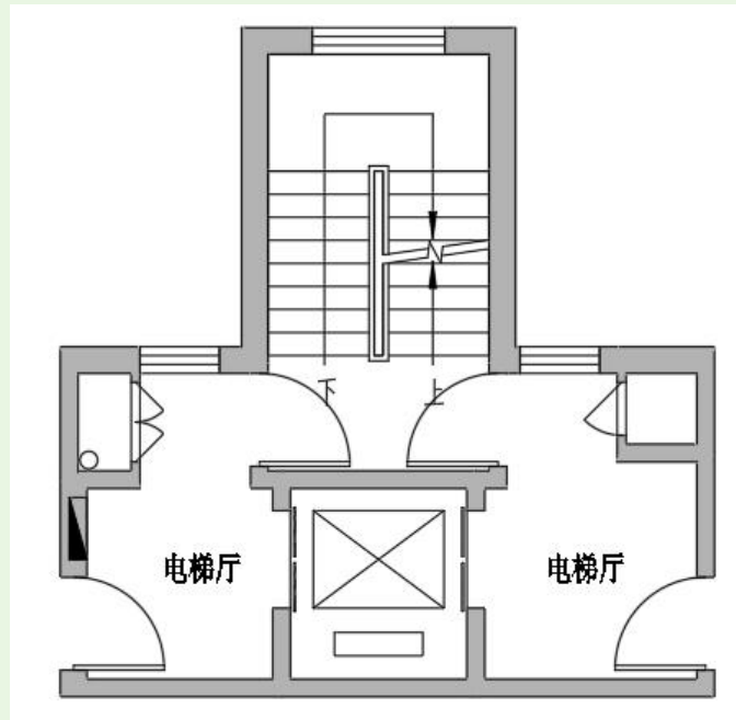
图 7.5 全明交通核、独立电梯厅
